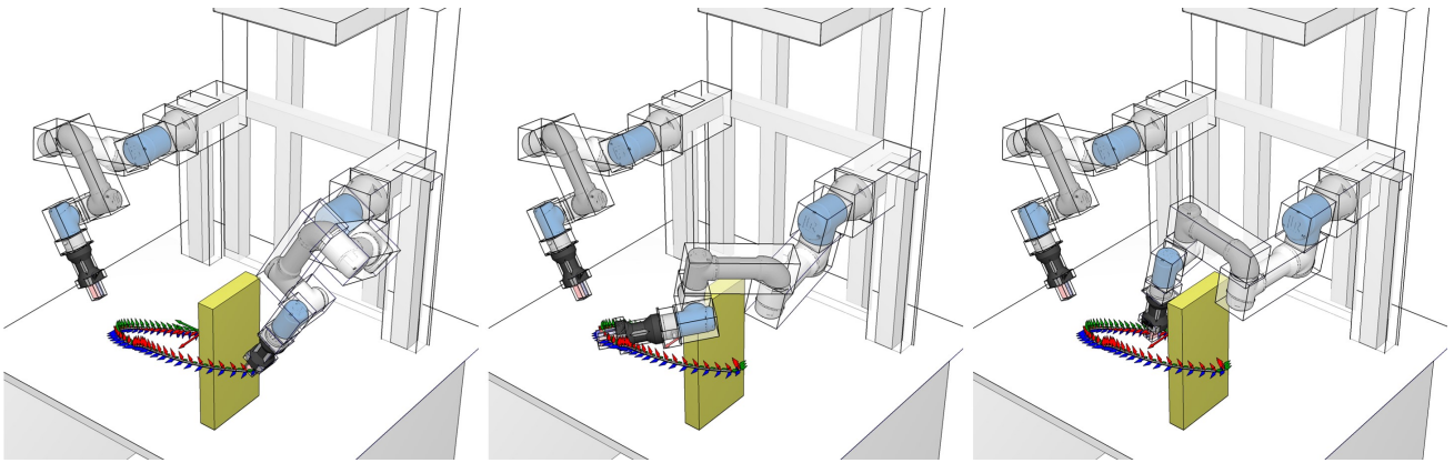
図 5: ur3_dual_planning.py の実行結果.
